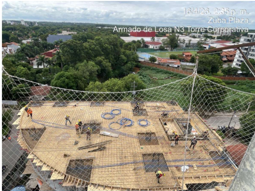
Avance Encofrado y Cargamento Losa N3
